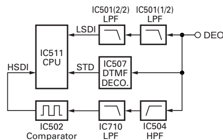
Fig. 14 Decode
